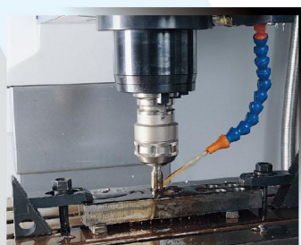
Rigid tapping
